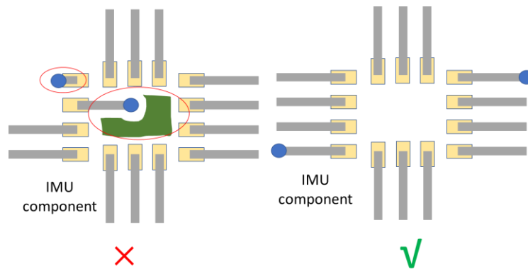
Figure 8. Avoid traces, vias and copper pour below IMUs
